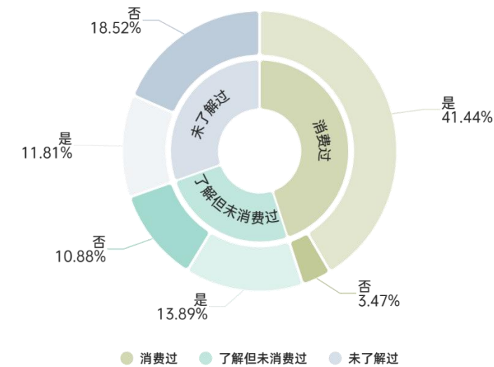
图 50 认知情况与购买意愿交叉分析图
